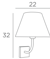
Lampshade ABA 1 o Ø 12-22-16 cm Lampshade code : 1111 + fabric code ↳ 23 cm
