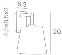
Lampshade EDFOU 1 o Ø 10-14-12 cm Lampshade code : 1125 + fabric code ↳ 16 cm
