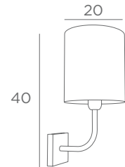
Lampshade ABA 2 cyl Ø 20-20-20 cm Lampshade code : 1205 + fabric code ↳ 25 cm
