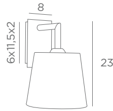
Lampshade EDFOU 2 o Ø 12-16-14 cm Lampshade code : 1126 + fabric code ↳ 19 cm
