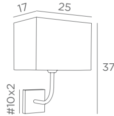
Lampshade ABA 2 rect □ 25x17-25x17-18 cm Lampshade code : 1412 + fabric code ↳ 23,5 cm
