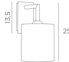
Lampshade EDFOU 2 cyl Ø 15-15-16 cm Lampshade code : 1204 + fabric code ↳ 18,5 cm
