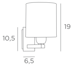
Lampshade RAMOSE 1 cyl Ø 13-13-14 cm Lampshade code : 1201 + fabric code ↳ 16,5 cm
