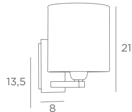
Lampshade RAMOSE 2 cyl Ø 15-15-16 cm Lampshade code : 1204 + fabric code ↳ 18,5 cm
