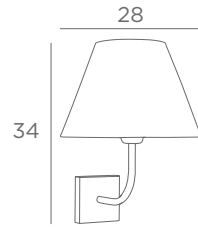
Lampshade ABA 2 o Ø 14-28-20 cm Lampshade code : 1112 + fabric code ↳ 29 cm
